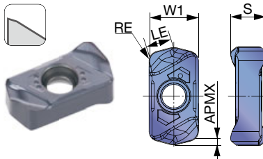
LNGU03ZER-MH (Robust cutting edges)
